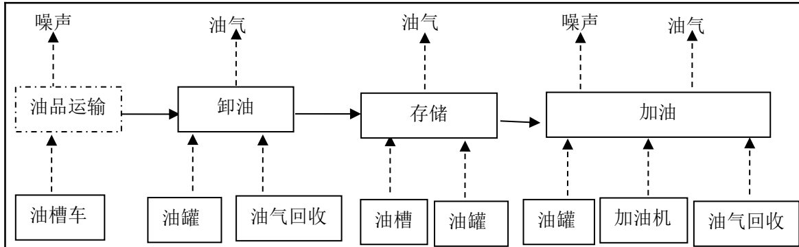
图 2-1 加油站汽、柴油加油工艺流程及产污环节图
